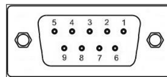
Figura 4: Conector de telemetria.
