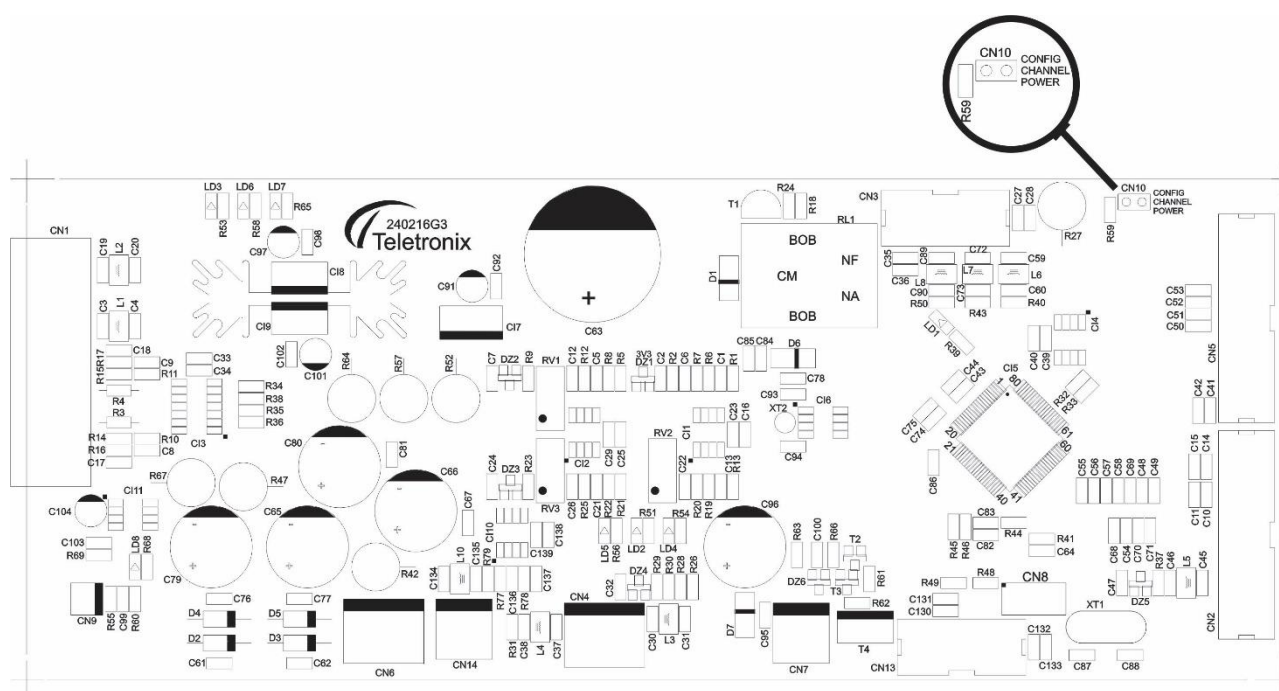
Figura 32: Jumper de configuração.
