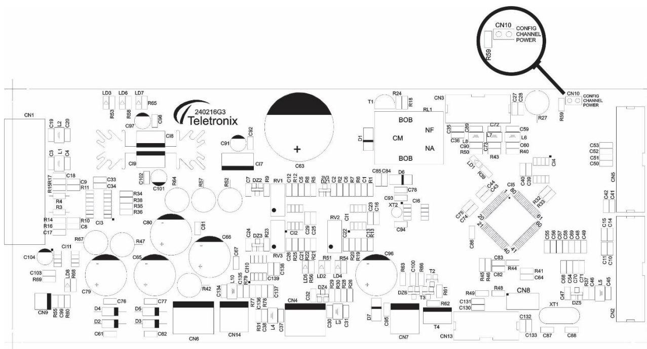
Figura 31: Jumper interno.
