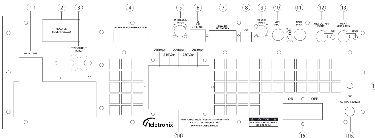
Figura 3: Painel traseiro.
