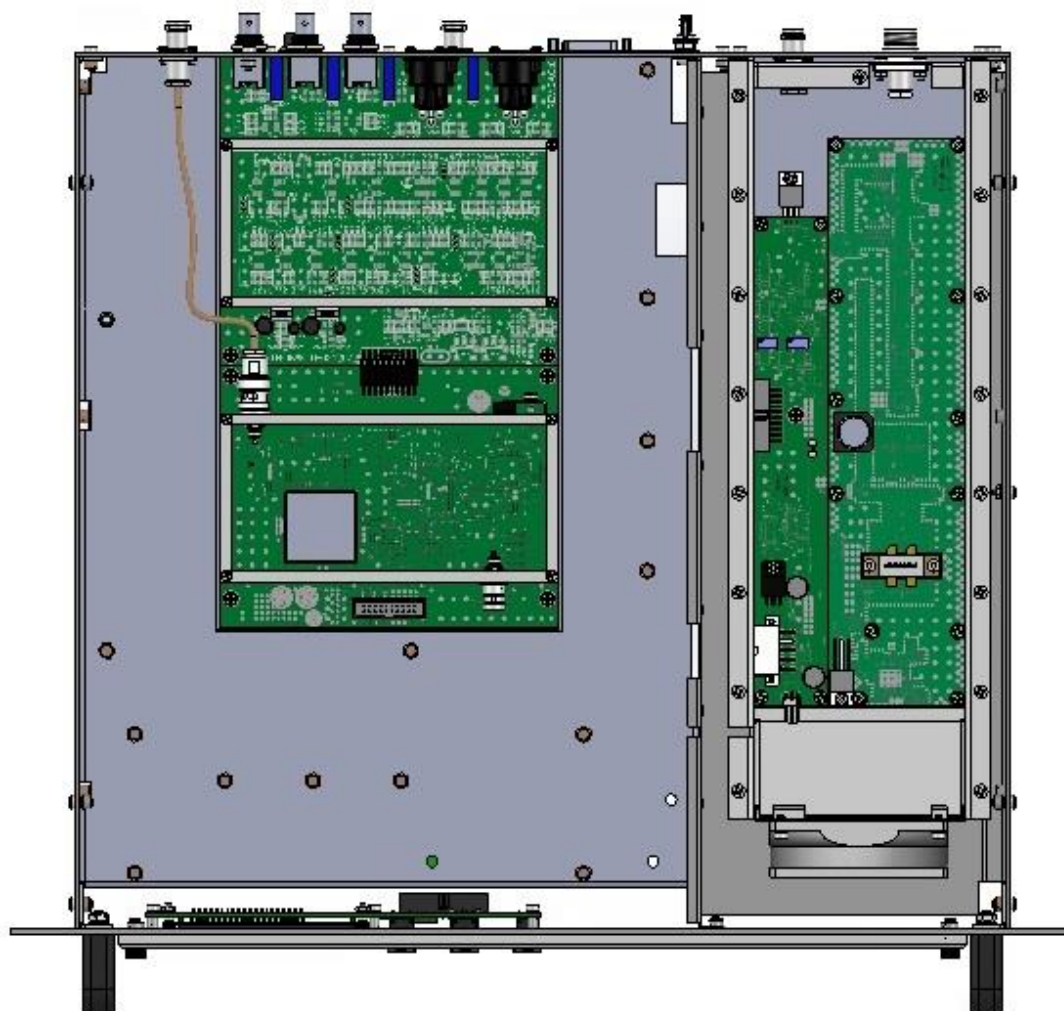
Figura 4: Vista superior do equipamento
