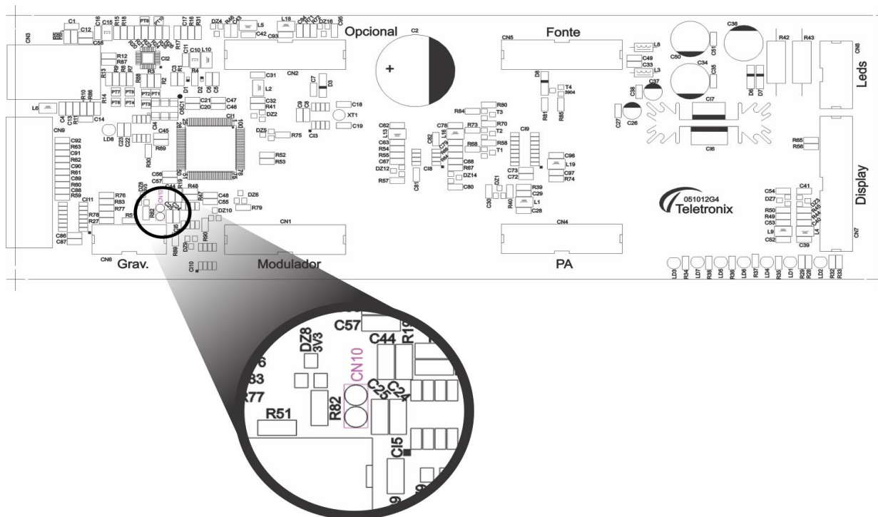
Figura 3: Localização do Jumper na PCI
