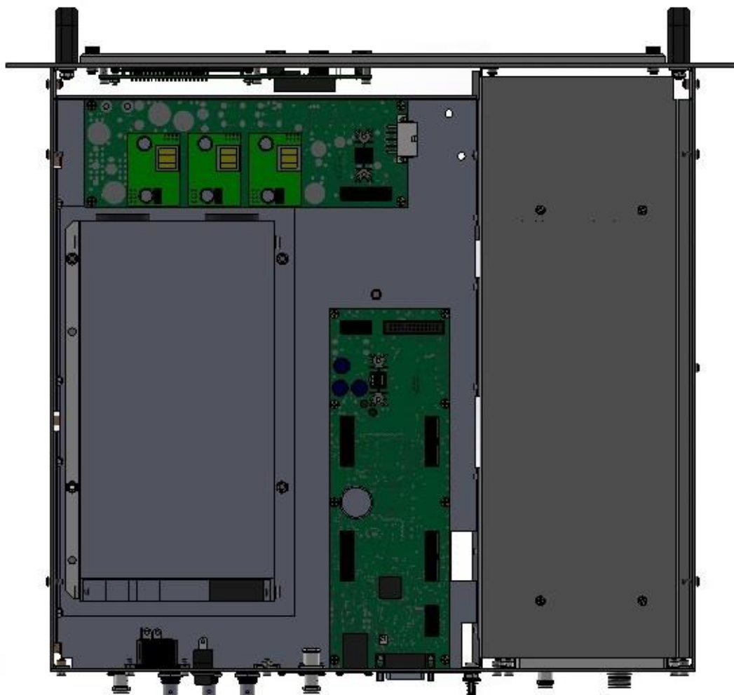
Figura 5: Vista inferior do equipamento
