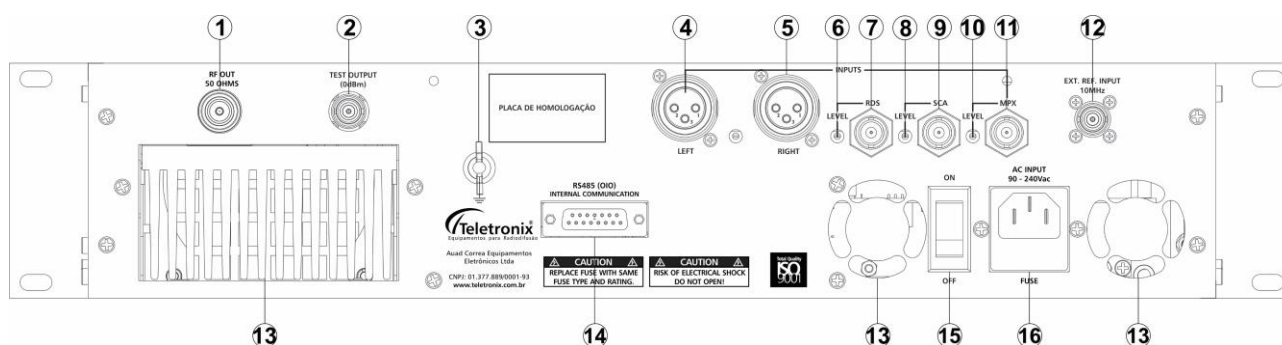
Figura 1: Painel Traseiro SP300
