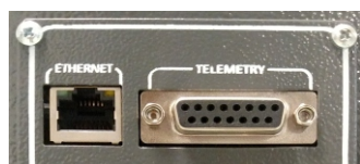
Detalhe para Comunicação RS232 e Ethernet
